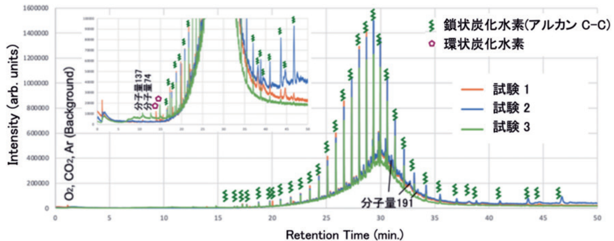
図5 GC/MS 熱脱着法によるトータル・イオン・クロマトグラム
