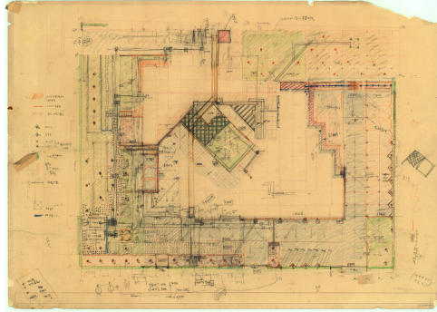
田崎美術館 Tasaki Museum of Art | 配置図 [外構図スケッチ] Site Plan [Landscape Sketch] | 1986
